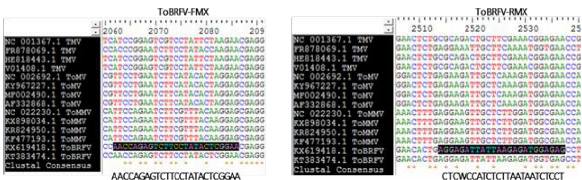
Figura 1. Región seleccionada para el diseño de los oligonucleótidos específicos para detectar a ToBRFV. A) Se consideraron los genomas de los Tobamovirus TMV, ToMV, ToMMV y ToBRFV.
